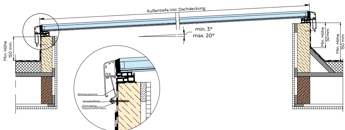
ClearSky 2-fach auf einem bautechnischen Aufsatzkranz. Tiefenquerschnitt.
