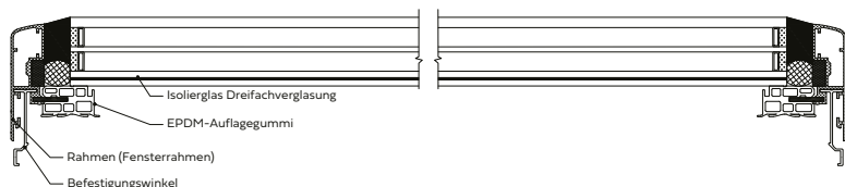
ClearSky 3-fach. Breitenquerschnitt.
